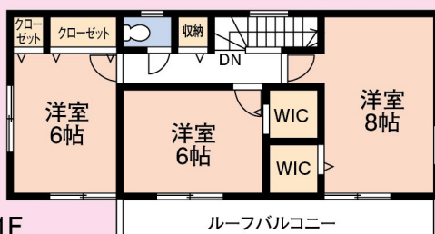
〈6号棟間取図〉
